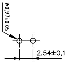
P.C.B. LAYOUT
