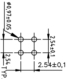
P.C.B. LAYOUT
